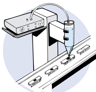
自动点胶机
